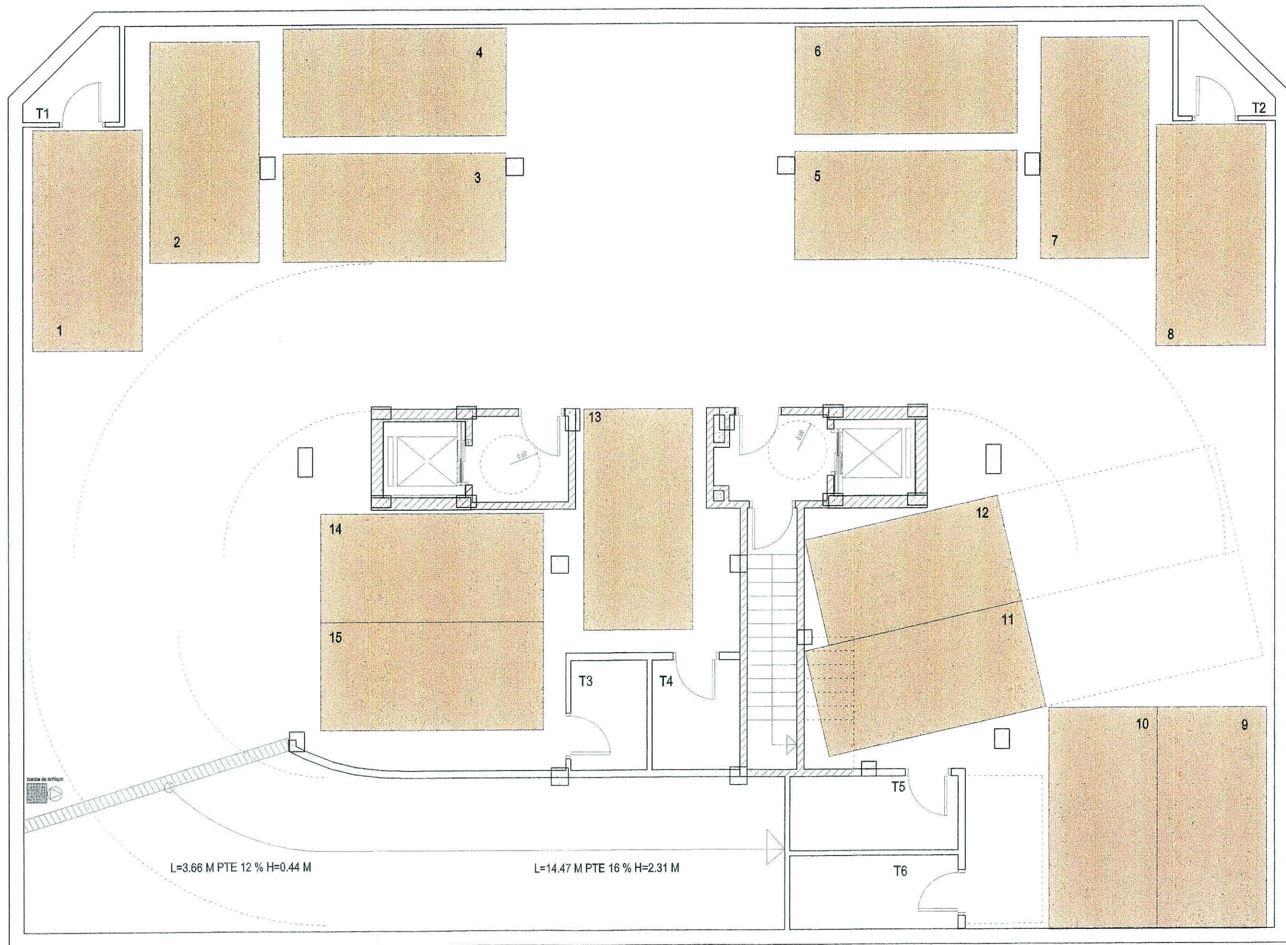
PLANTA SÓTANO E: 1/75
